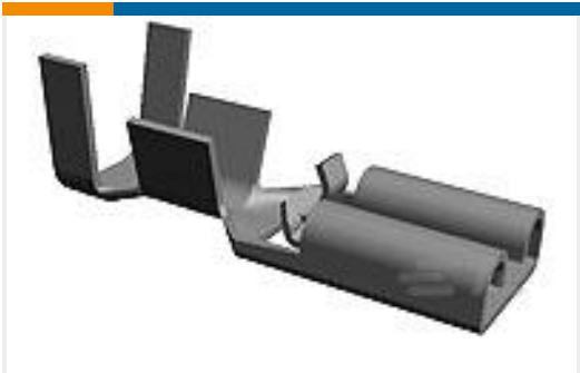
TE 产品编号1217113-2 187 PL MKIII REC. 22-18AWG TPBR
