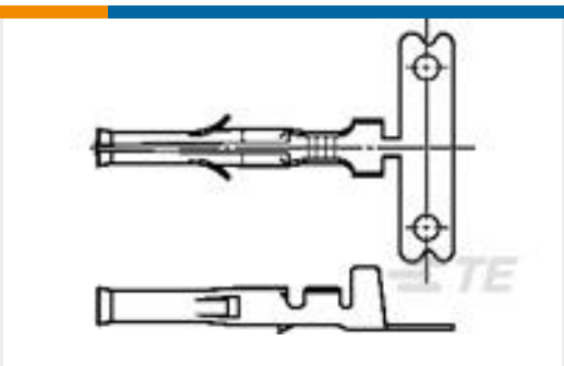
TE 产品编号350628-5 .062 COMM P&S SOK AUNI/BR
