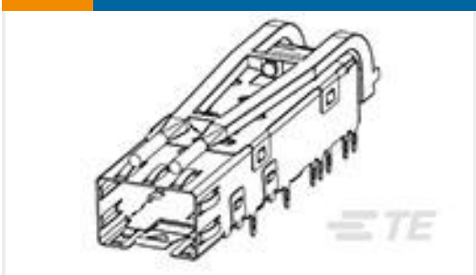
TE 产品编号2170614-1 cage assy, 20 press fit, sfp w
