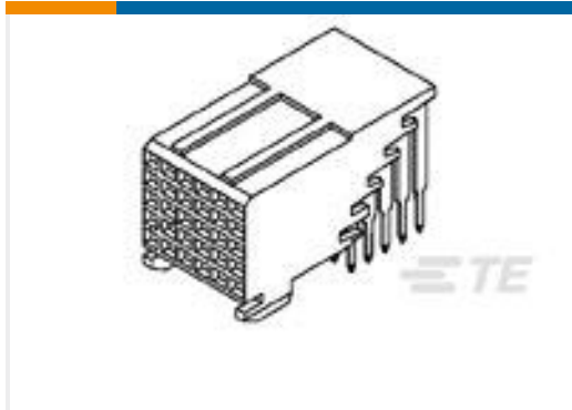
TE 产品编号223007-2 FB-5R, ASY, 060, SIG, REC, SL, 3.53
