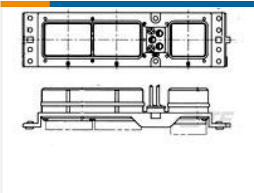
TE 产品编号3-208973-5 ASSY,PLUG,SZ2,ARINC 600
