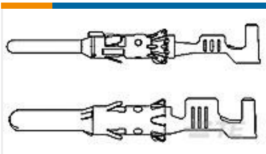
TE 产品编号1703018-1 DIA 1.5MM CONTACT PIN,LP
