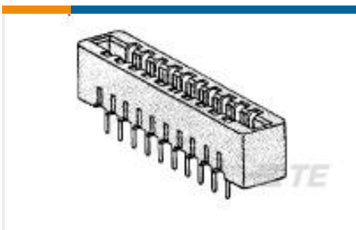
TE 产品编号2-530666-3 CONN LOW PRO 12 POS 156X200C/L
