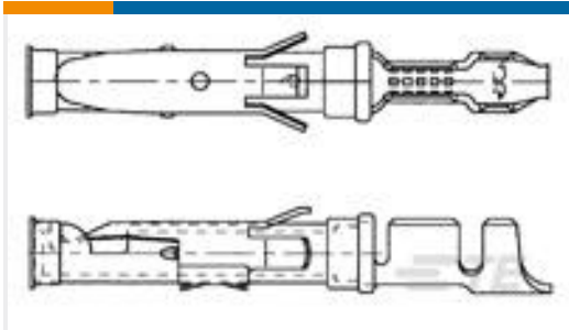
TE 产品编号 163083-2 .062 DIA SOC ASS 3+
