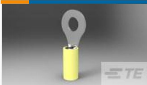
TE 产品编号 165034 PIDG RING 12-10 1/4
