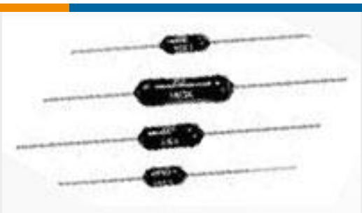
TE 产品编号1879666-7 H8 154K 0.1% 15PPM
