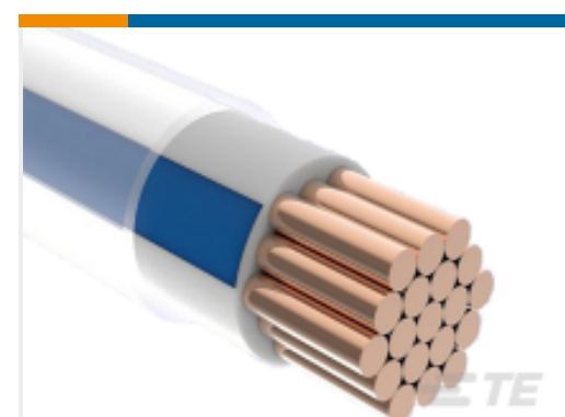
TE 产品编号6171143001 ACW0219-0.75-26(NS)
