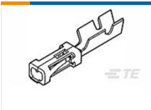
TE 产品编号167301-4 MOD-4 REC.CONT.SCP
