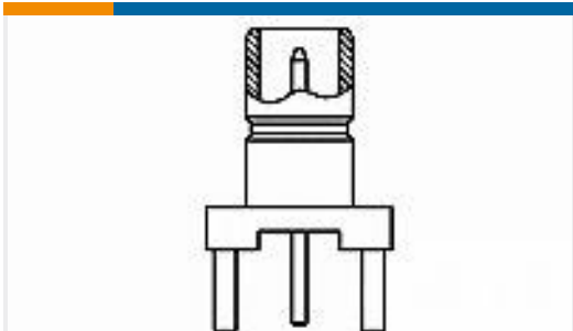
TE 产品编号415504-4 JACK,PCB,MINI-SMB VERT 75 OHM
