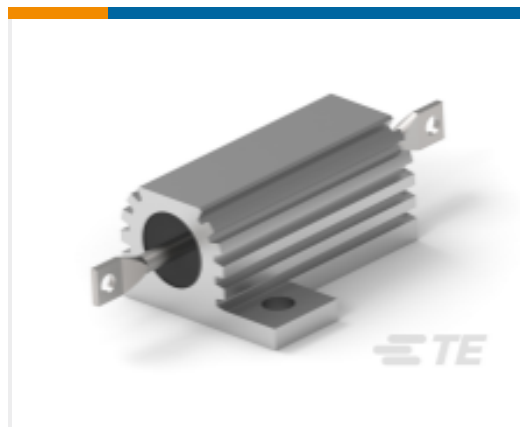
TE 产品编号1-1879073-0 功率电阻器：铝壳体，75 瓦特
