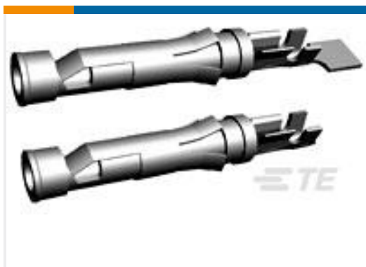
TE 产品编号1-66360-3 III+ SKT, 18-14, TIN, SMPACK
