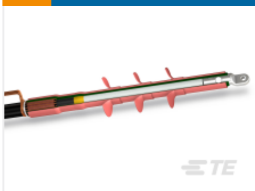
TE 产品编号F77770-014 POLT-24C/1XO
