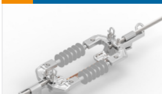
TE 产品编号1710730-3 35kILD-L-FRAME-KS9C
