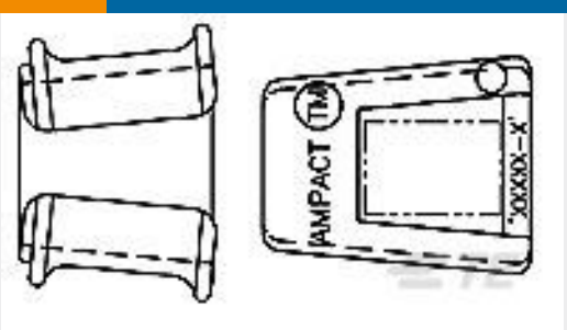
TE 产品编号602380-6 AMPACT Tap 350-4/0
