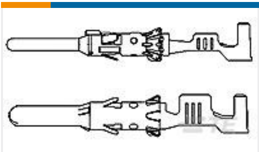
TE 产品编号1-929964-0 2,5MM STIFTKONTAKT
