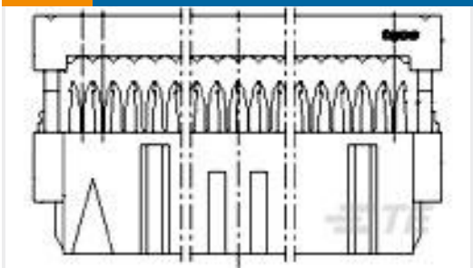
TE 产品编号1-215882-6 16 WAY GREY MK II RECP
