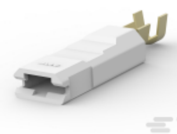
TE 产品编号5-520963-1 ULTRA POD: 直形, 母端组件, 无镀层, 0.250 英寸
