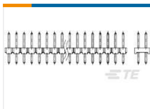
TE 产品编号1734508-6 AMPMODU,2.0MM, HDR, VRT MT, 8u" AU, 6P
