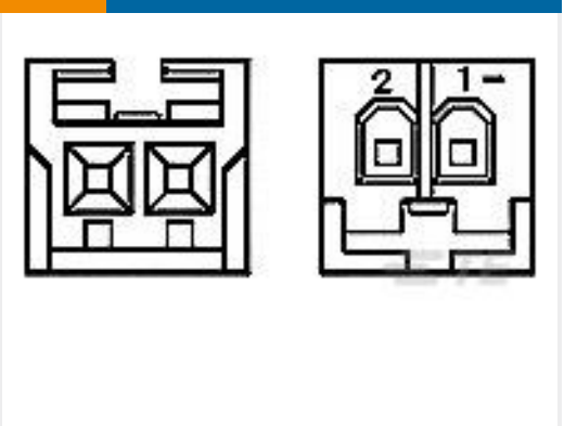
TE 产品编号2-172486-2 2P REC HSG CRIMP EI SER BLACK
