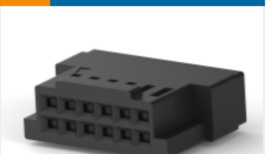
TE 产品编号3-88179-2 2.54mm FFC 连接器母端外壳
