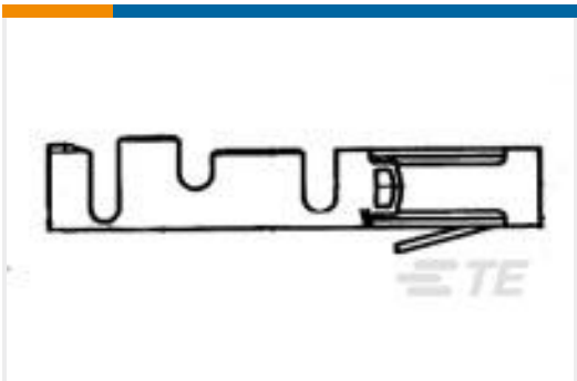
TE 产品编号182206-2 MOD 2 TERMINAL
