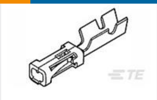
TE 产品编号166310-3 MOD-5 REC.CONTACT
