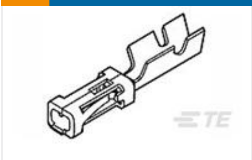
TE 产品编号141603-4 MOD-4 REC.CONTACT
