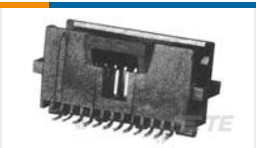
TE 产品编号104549-3 24 SYS50 SURFMNT HDR DRST SHRD
