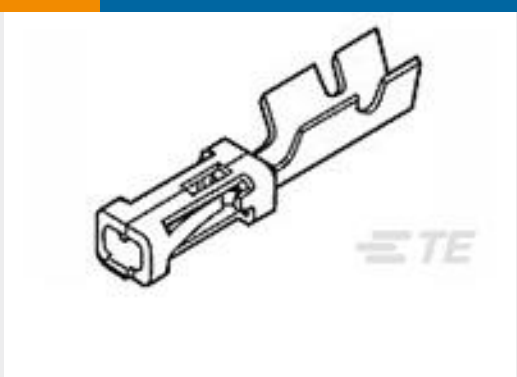
TE 产品编号102920-2 MOD IV RECP LP
