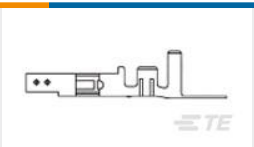
TE 产品编号1586317-4 VAL-U-LOK SKT PHBZ AU 26-22 LP
