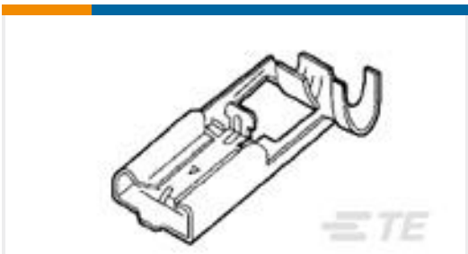
TE 产品编号172795-1 PL 312 FLAG REC 20-14 0.32 X 24.9 PTPBR
