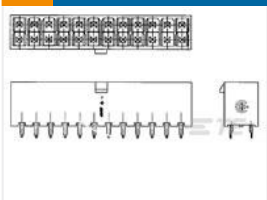
TE 产品编号1-1586768-4 14P VERT HDR VAL-U-LOK GW
