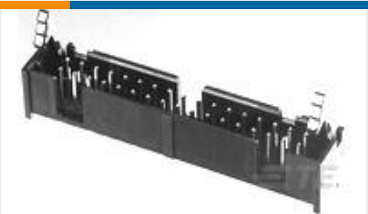
TE 产品编号104313-2 014 LOPRO HDR SP 30DP LATCH
