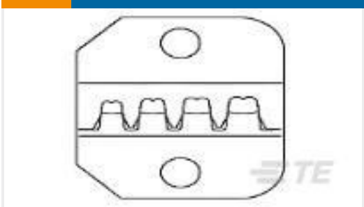
TE 产品编号1424050-1 PREMIUM SDE DIE BNC
