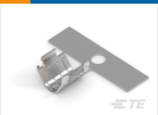
TE 产品编号2298509-2 MINI COAX SHIELD CRIMP FERRULE RG174
