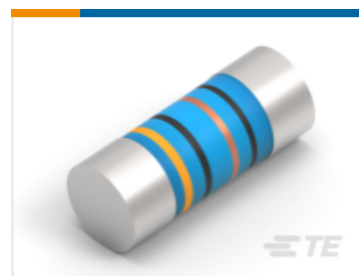
TE 产品编号1-2176315-2 MELF SMA_A 820R 0.1% 15PPM 0204 0.4W
