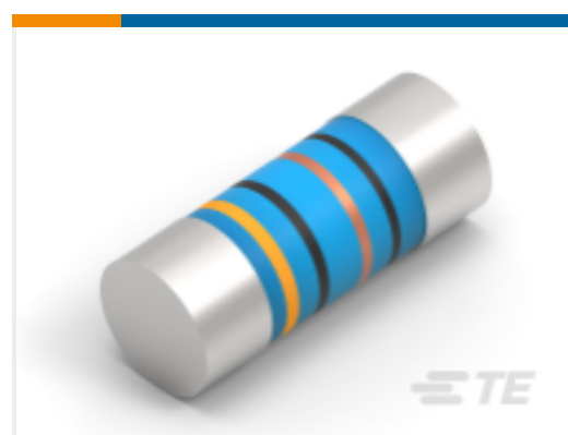
TE 产品编号1-2176315-0 MELF SMA_A 560R 0.1% 15PPM 0204 0.4W
