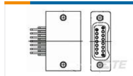
TE 产品编号2-1589483-6 STL051L2HN = SMT CONN
