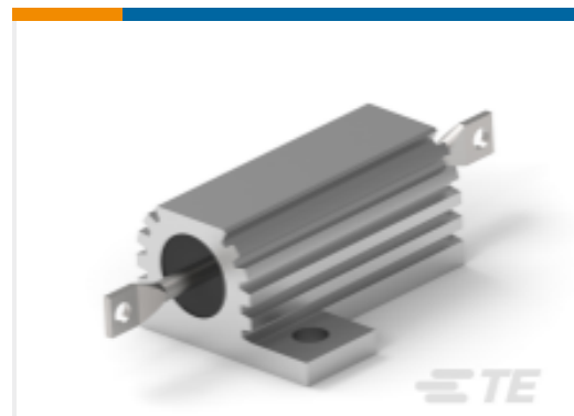
TE 产品编号1-1879073-0 功率电阻器：铝壳体，75 瓦特
