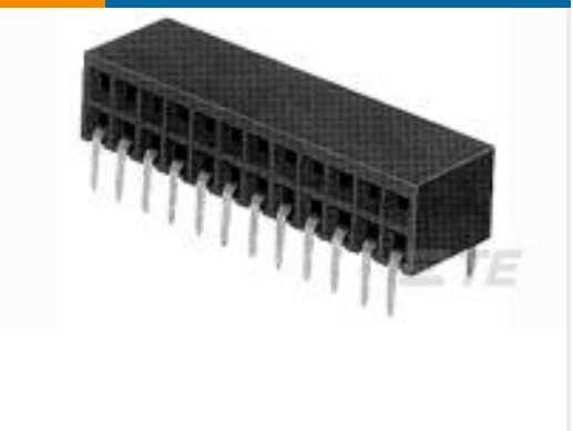
TE 产品编号1-87962-9 40 MODII HORZ DR CE 100CL/115
