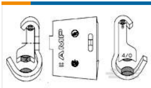
TE 产品编号83623-4 MINIWEDGE,LRG SL,2/0-#4
