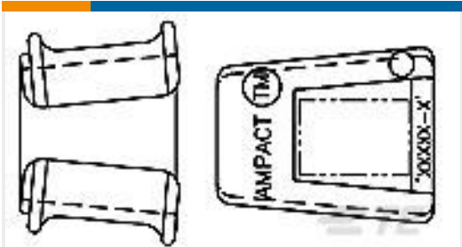
TE 产品编号602283-1 AMPACT AI Tap 2-2,1/0-4
