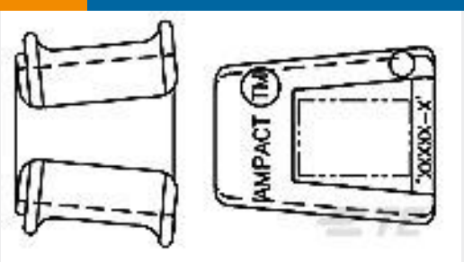
TE 产品编号602380-7 AMPACT Tap 350-350
