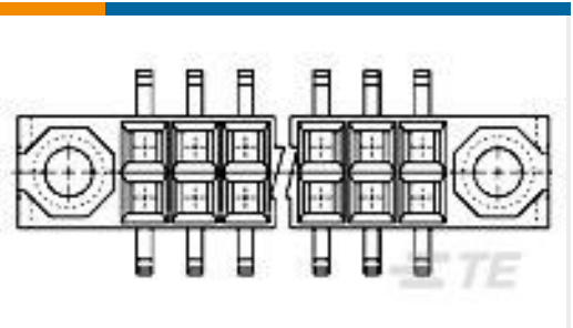
TE 产品编号534286-9 26 MODIV VERT DR 100CL/SFMNT
