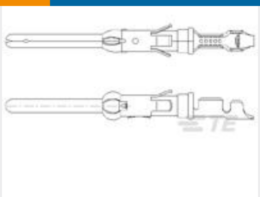
TE 产品编号163085-8 .062 DIA PIN ASS 3+
