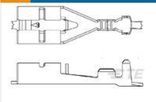
TE 产品编号1380087-1 PL MKIII L.I.F 250 REC 0.5-1.0 MM2 BR
