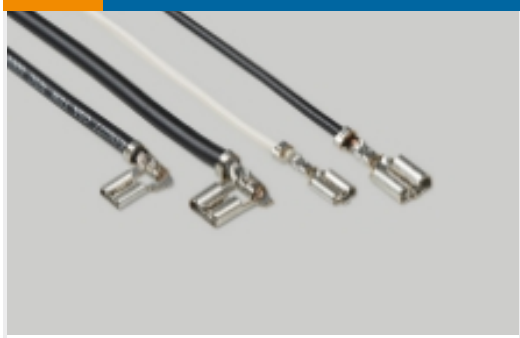
快速断开(38)
