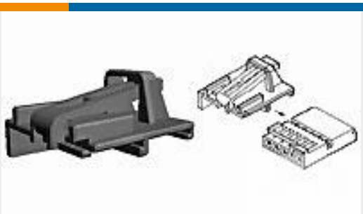
TE 产品编号1418776-2 COVER,MQS,5 POS.
