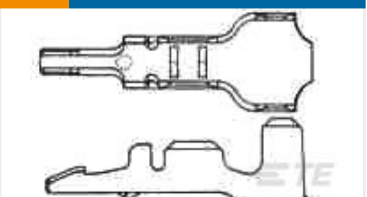
TE 产品编号170197-2 MINI AMP-IN 24-20 AWG
