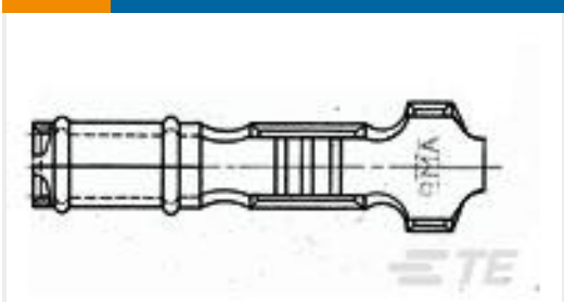
TE 产品编号170137-1 .058 DIA P.C.B REC LP
