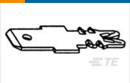
TE 产品编号1601018-2 131-044-014=TAB,187X020,STDSMZ
