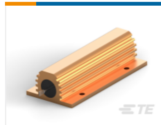
TE 产品编号3-1625999-6 功率电阻器：铝壳体，HSC
