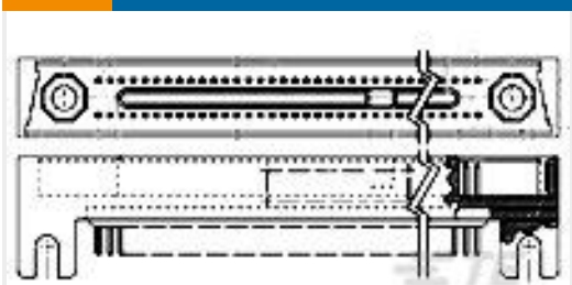
TE 产品编号1057341-1 3080 2240 00
