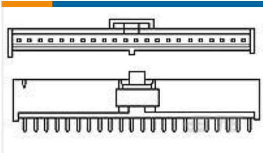
TE 产品编号3-1888291-3 FPH-2021G=FLXPAC HDR P 20 ST L
