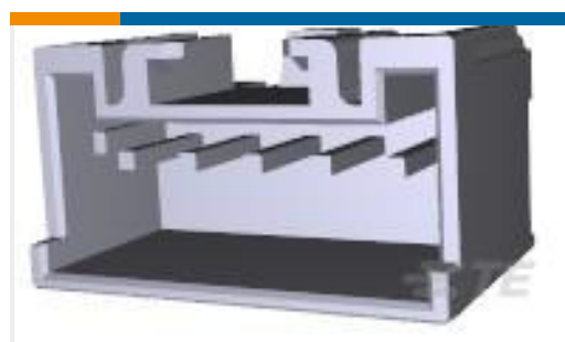
TE 产品编号917783-2 2.5 S.D.L STD 5P HDR ASSY
